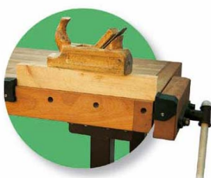
Spannen mit Steckspannbacken – vor bzw. auf der Werkbank
